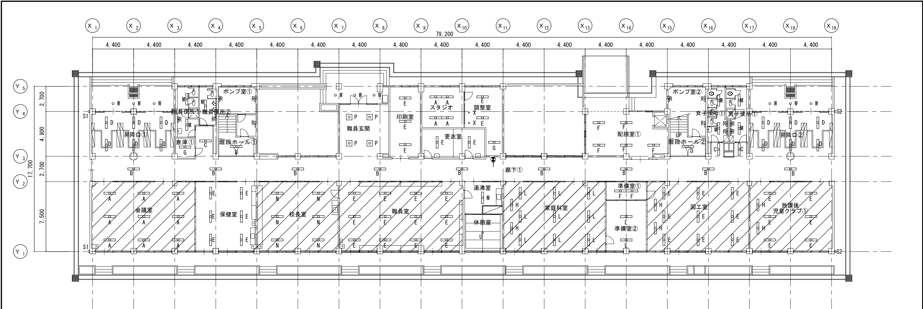
1 階 平 面 図
