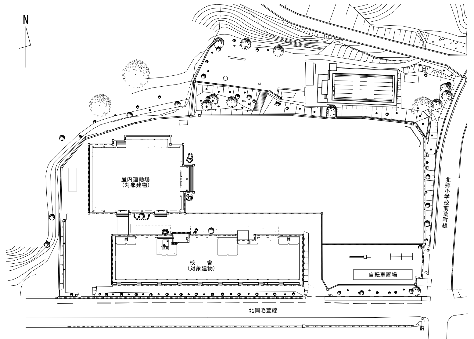
配置図 S=1/600
