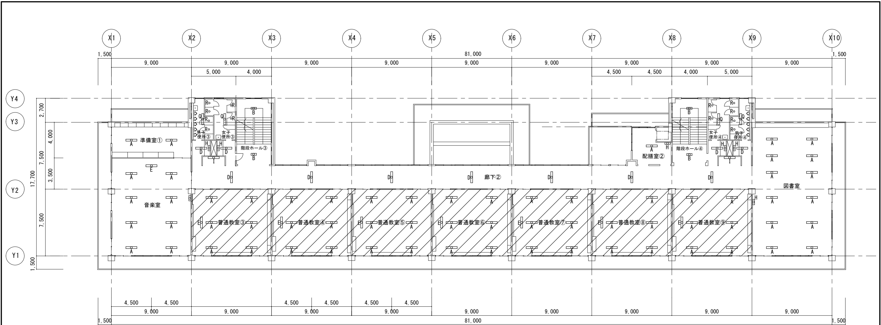
2 階 平 面 図
