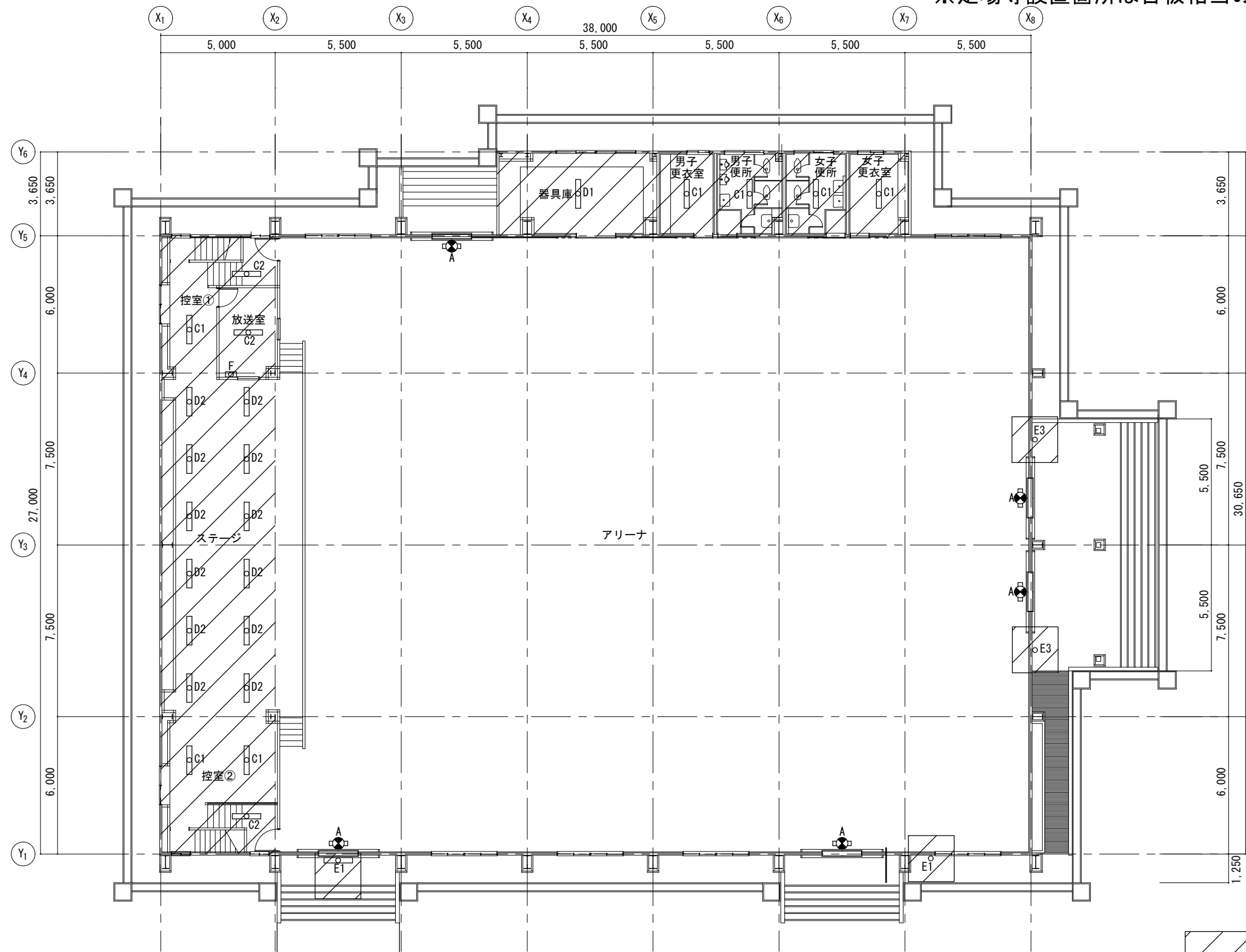
1 階 平 面 図
