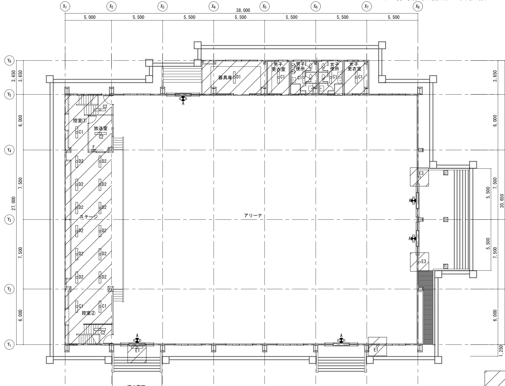
1 階 平 面 図
