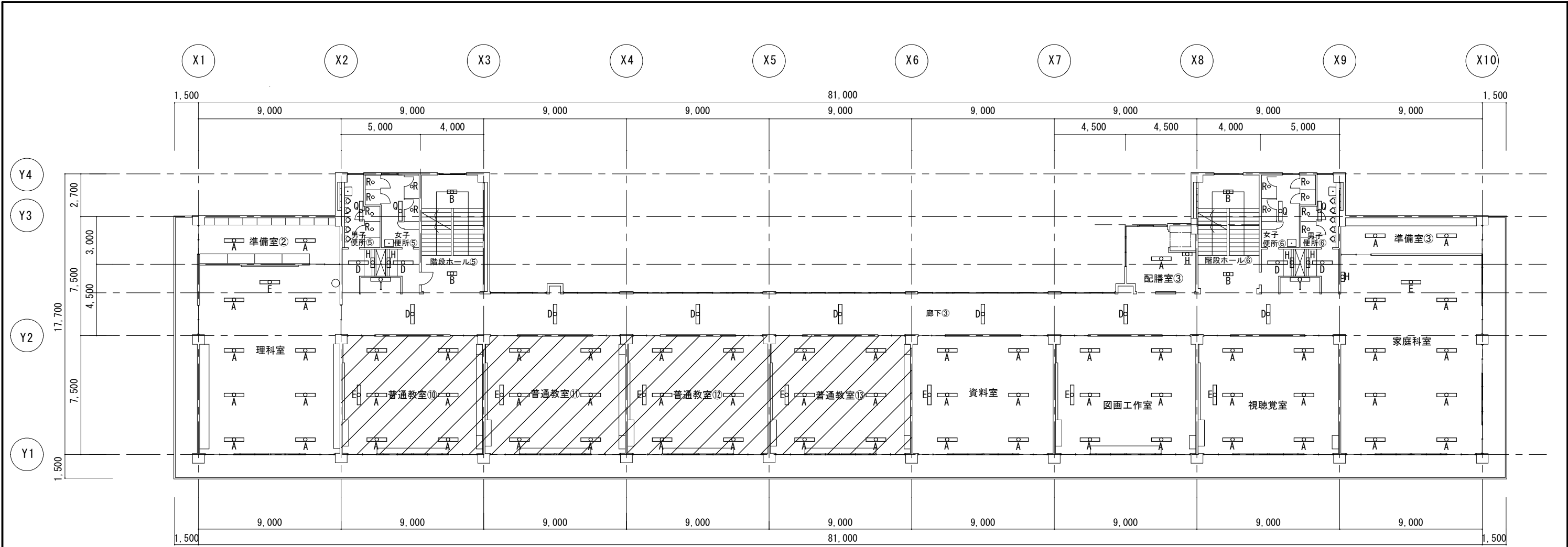
3 階 平 面 図
