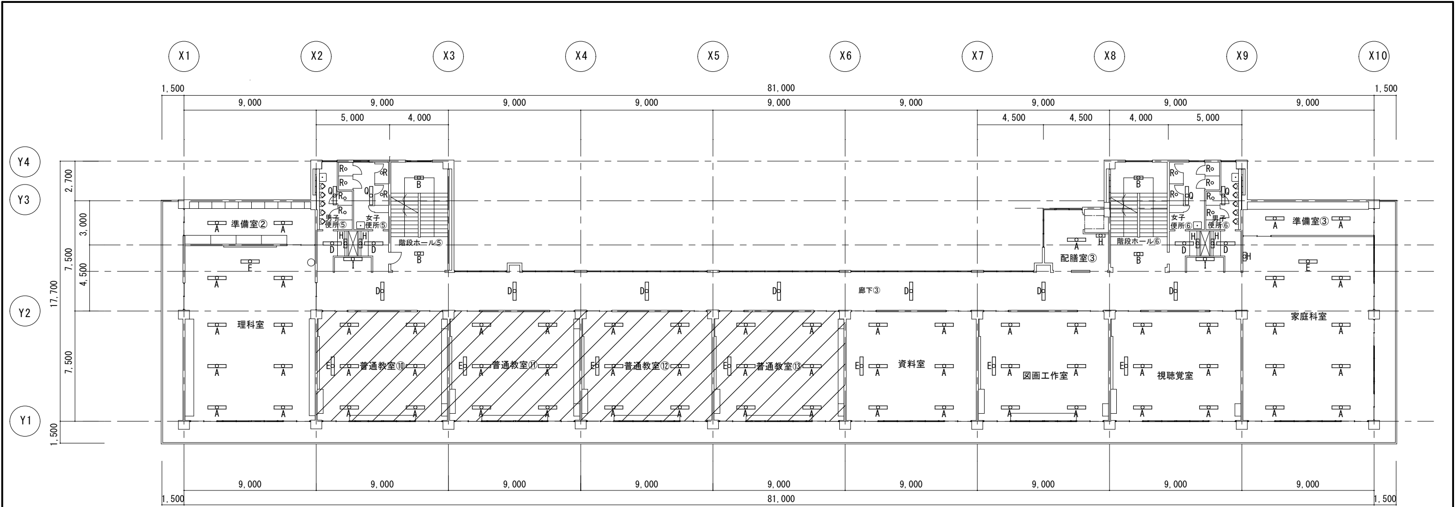
3 階 平 面 図
