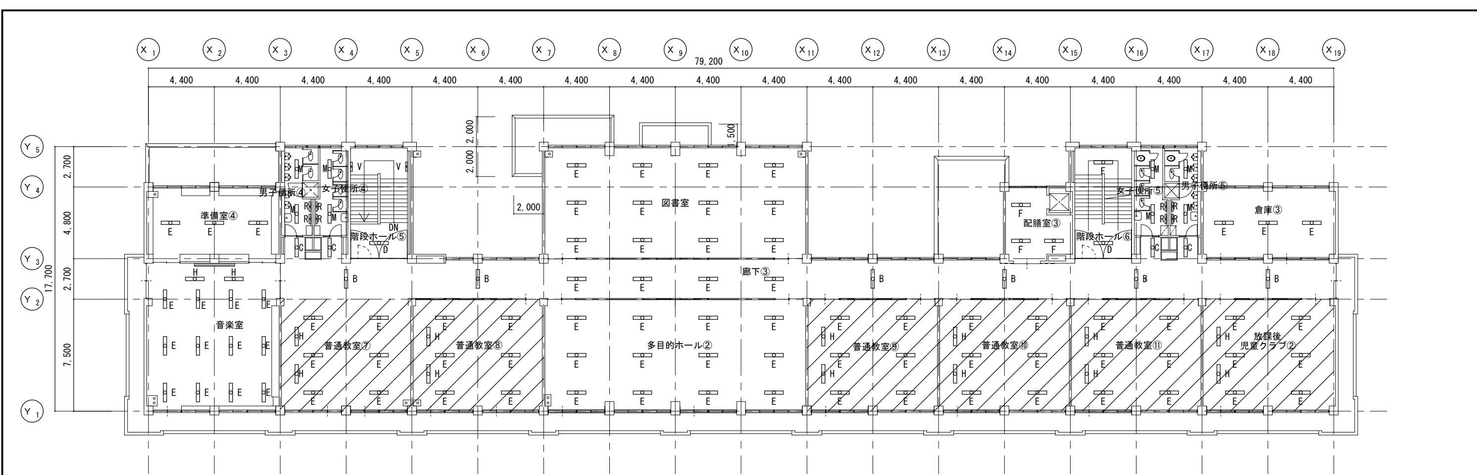
3 階 平 面 図
