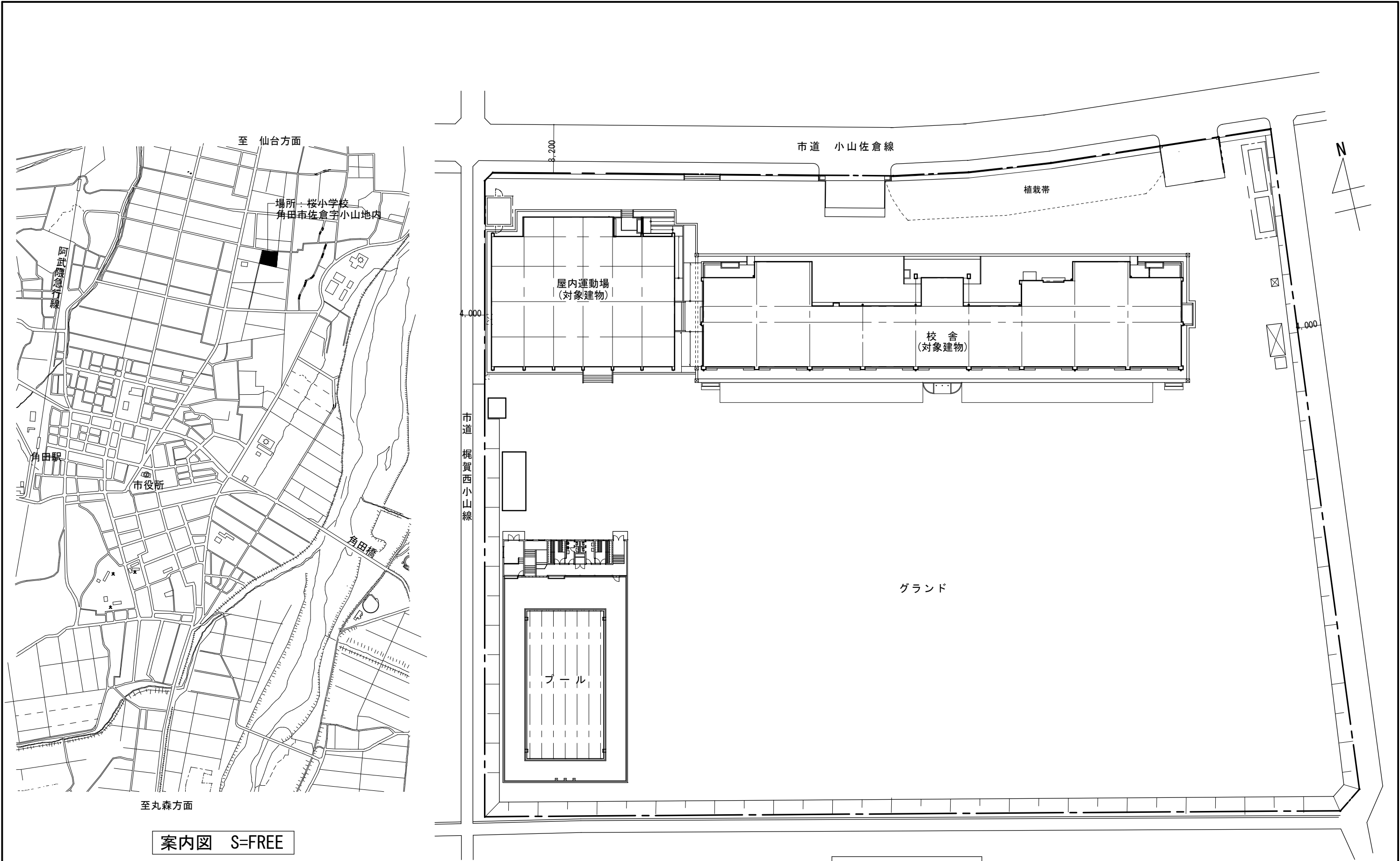
配置図 S=1/600
