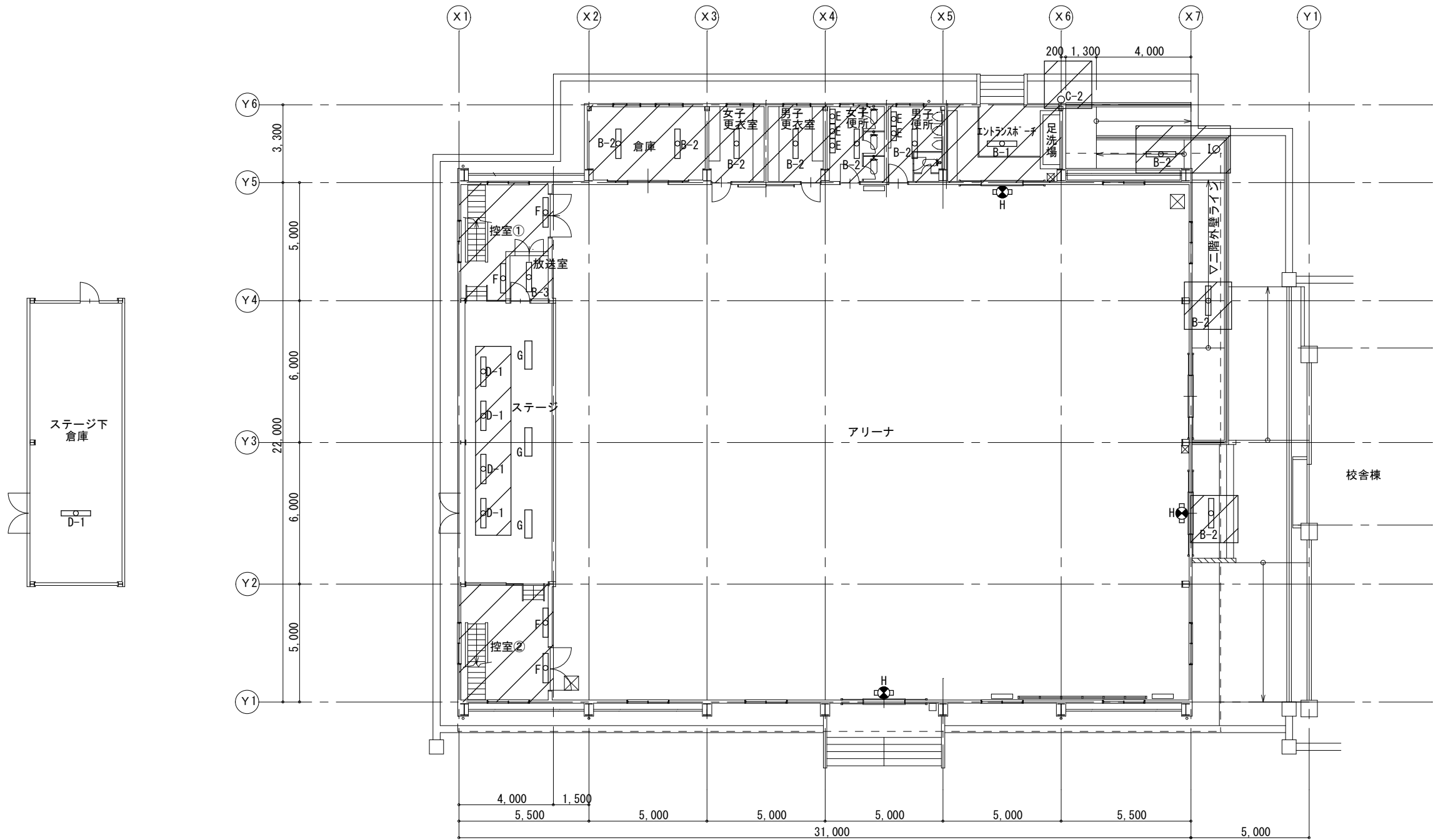
1 階 平 面 図
