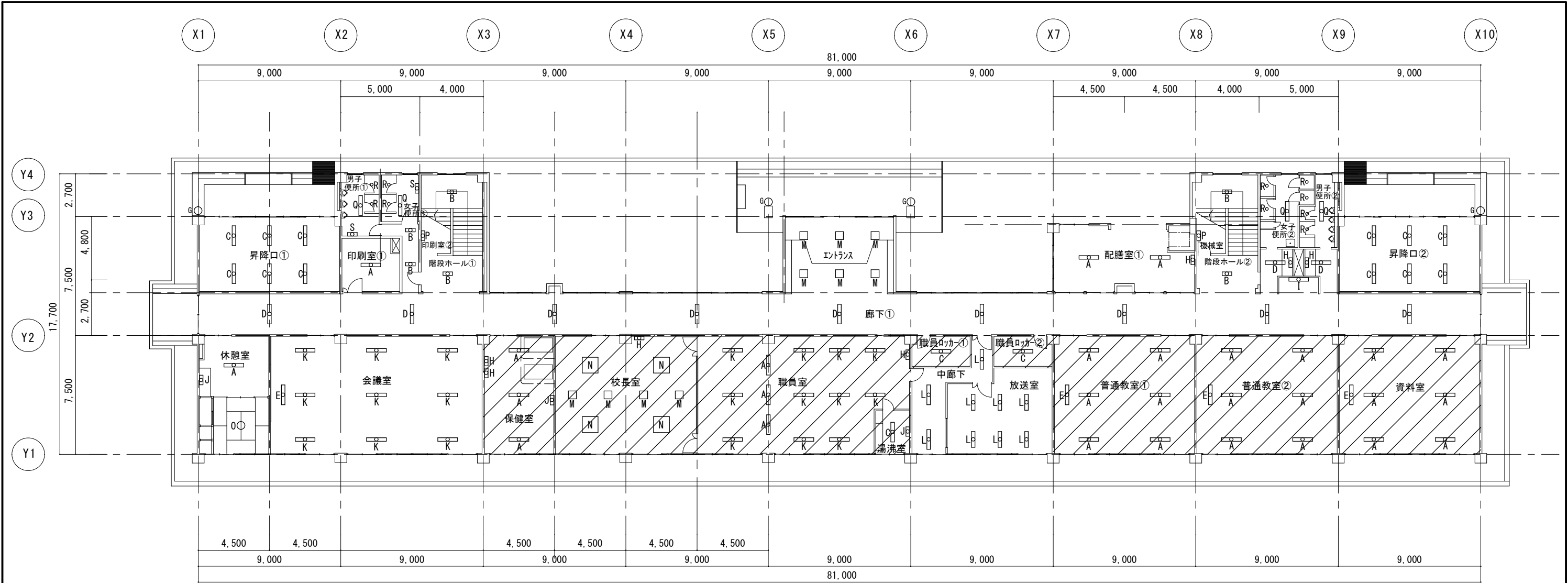
1 階 平 面 図
