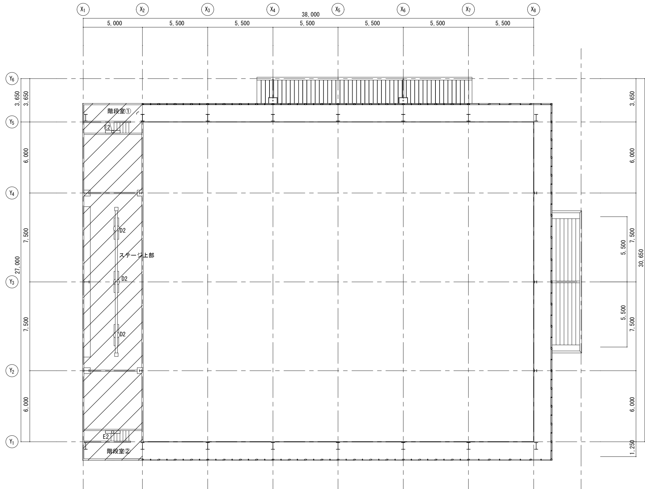
2 階 平 面 図
