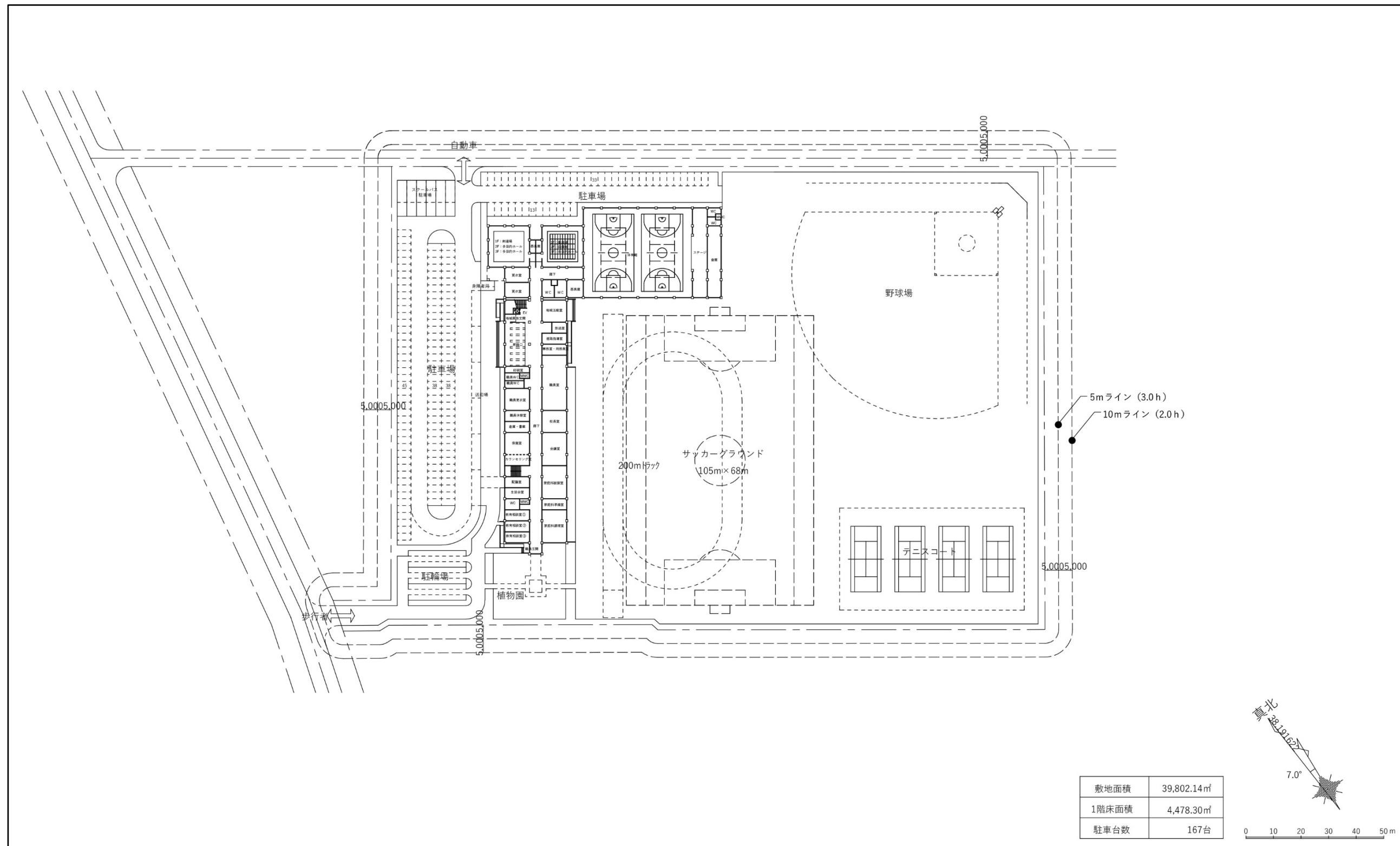
图 1-10-2 L 字型校舍 配置图
