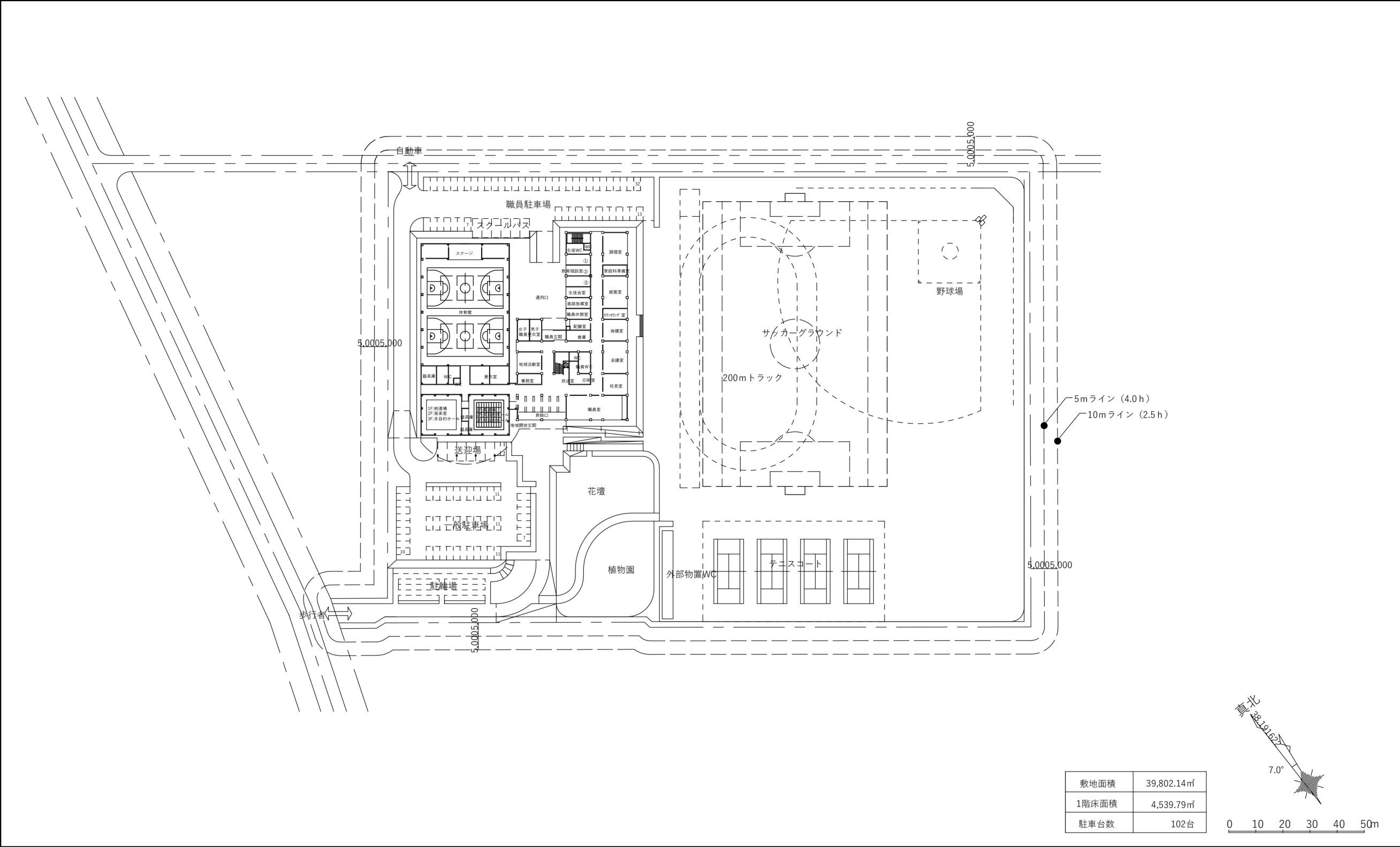
図 1-10-4 集中型校舎 配置図
