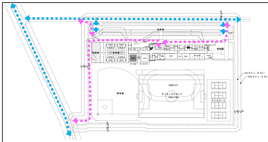
図 1-9-4 北側配置案
