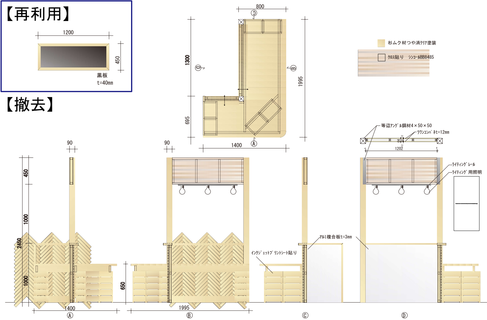
改修前 什器立面図 1 (参考図) A1:1/20 , A3:1/40 改修前 什器立面図 2 (参考図) A1:1/20 , A3:1/40
