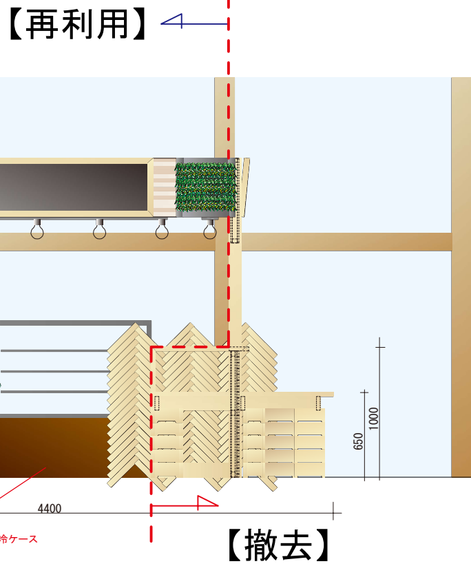
改修前 什器立面図 1 (参考図) A1:1/20 , A3:1/40 改修前 什器立面図 2 (参考図) A1:1/20 , A3:1/40
