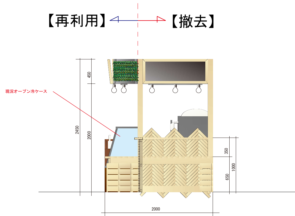
改修前 什器立面図 1 (参考図) A1:1/20 , A3:1/40 改修前 什器立面図 2 (参考図) A1:1/20 , A3:1/40
