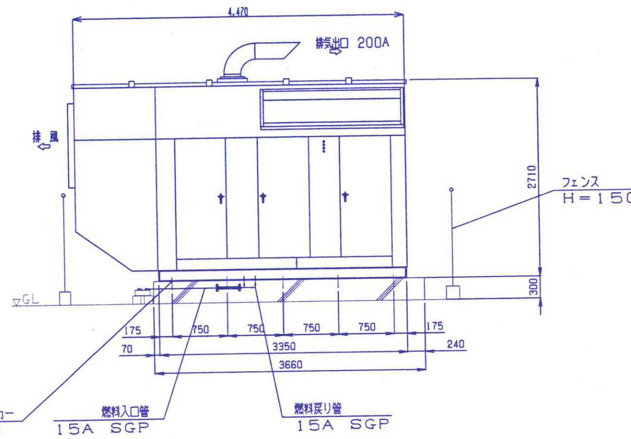
B-B' 断面図 S=1/50
